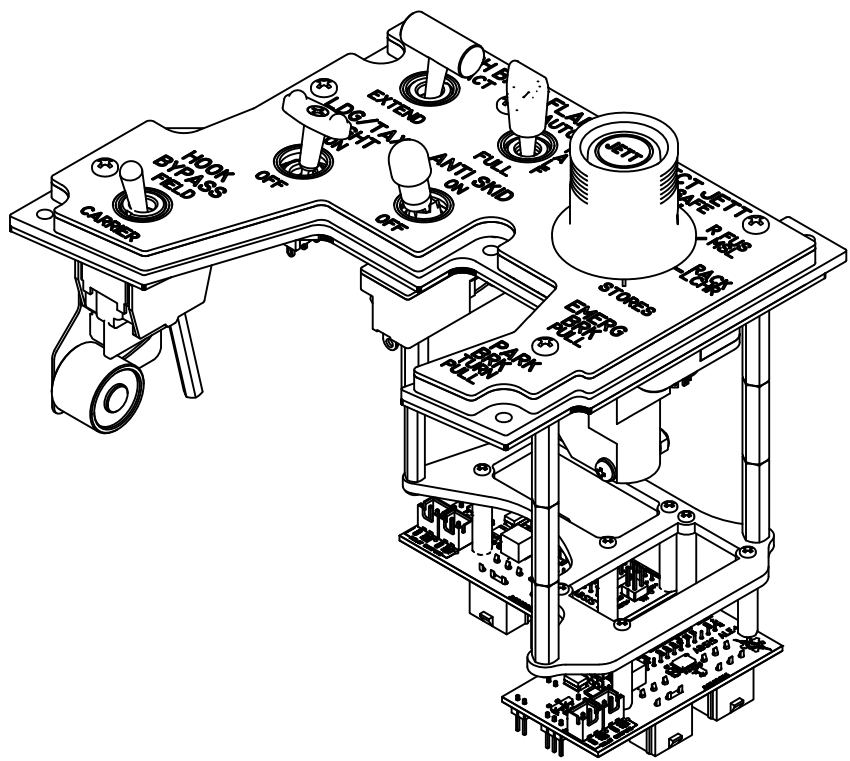
-1 ISO
